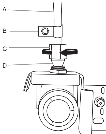
A. Tubería de cobre B. Abrazadera en "P" C. Tuerca de compresión D. Manga de compresión
