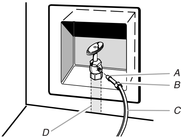
A. Bague B. Écrou C. Canalisations en cuivre (jusqu'au réfrigérateur) D. Canalisations d'alimentation en eau du domicile (1/2 po minimum)
